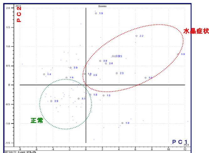
第1主成分と第2主成分のスコアプロット
